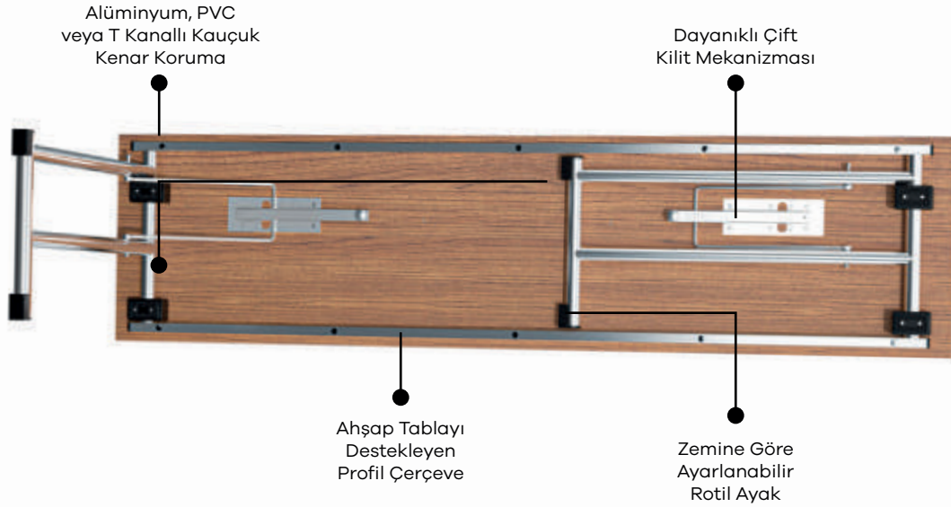
Alüminyum Kenar
